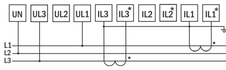
Рис. 10 – Подключение трансформаторов тока (трехфазная цепь без нейтрали)
