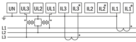
Рис. 14 – Подключение трансформаторов тока и напряжения (трехфазная цепь без нейтрали)
