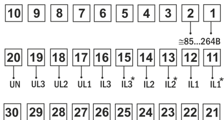
Рис. 6 – Клеммы подключения P99-M(AVFC)-3-0.5
