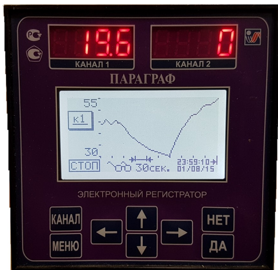
Рис.2.1. Лицевая панель прибора с ЖК дисплеем
