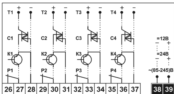
Рис.2.5 Схема включения ЦАП, кнопок и исполнительных устройств
