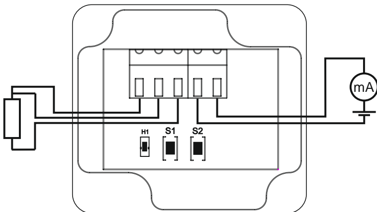
Рис. 5.1. Схема подключения датчика а) Спрут Т-02, Т-022 б) Спрут Т-026
