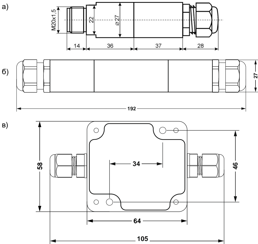
Рис.2.1 Измеритель-преобразователь а) СПРУТ Т-02, б) СПРУТ Т-022 в) СПРУТ Т-026
