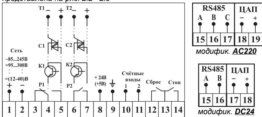
Рис. 2.2. Схема подключения прибора ( кроме исполнения H57 )
