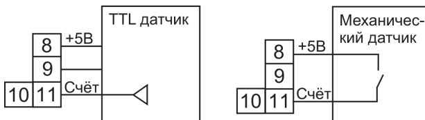
Рис. 2.4 Подключение датчиков
